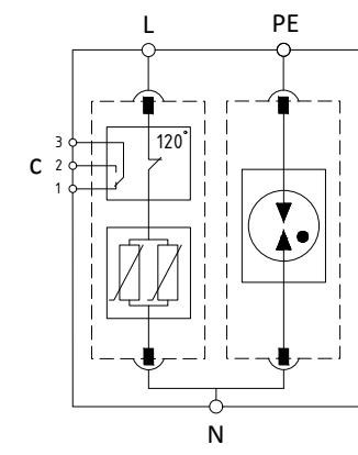
Принципиальная схема
